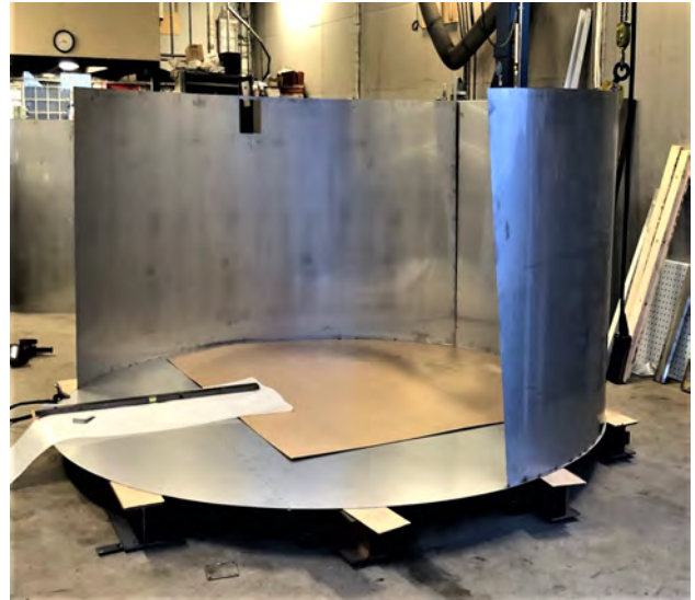
Altaan pystyseinät hitsauksessa
